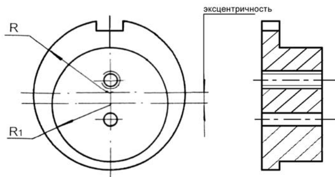
Рис. 6 – Эксцентрическое основание
