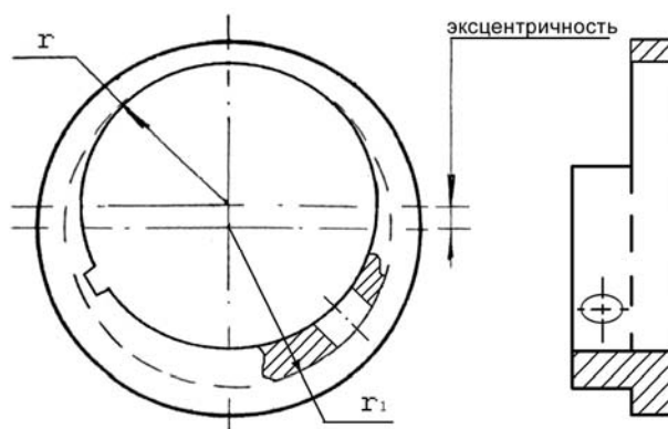
Рис. 7 – Эксцентрическое кольцо
