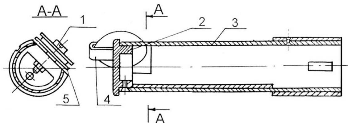
Рис. 3 – Второе (подвижное) колено мачты 1 – болт; 2 – основание; 3 – труба; 4 – скоба; 5 – ролик
