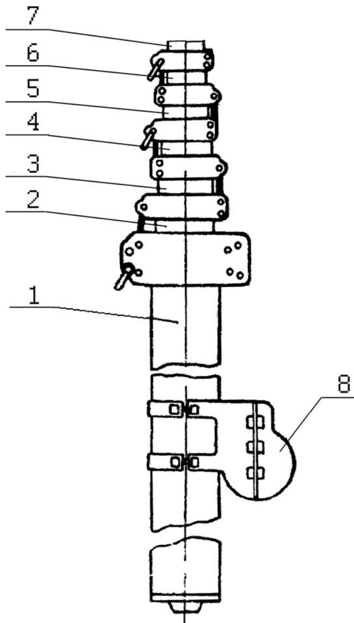
Рис.1 – Телескопическая мачта
